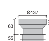
A WC - Stos, Centrisk RSK 310 66 84 NRF 619 66 72
