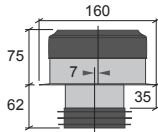
A GAS - WC 7 Utan huv, Excentrisk 7 mm RSK 310 67 03 NRF 56 884 21
