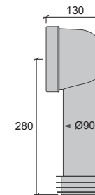
A + K3 WC - Stos, Universal RSK 310 67 20 NRF 619 66 71
