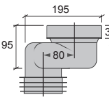
A + K2 WC - Stos Offset 80, Excentrisk 80 mm RSK 310 66 79 NRF 619 66 54
