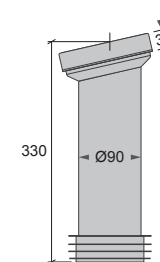
A + K3 WC - Stos, Vinklad RSK 310 67 23
