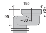
A + K2 WC - Stos Offset 80, Excentrisk 80 mm RSK 310 66 79 NRF 619 66 54
